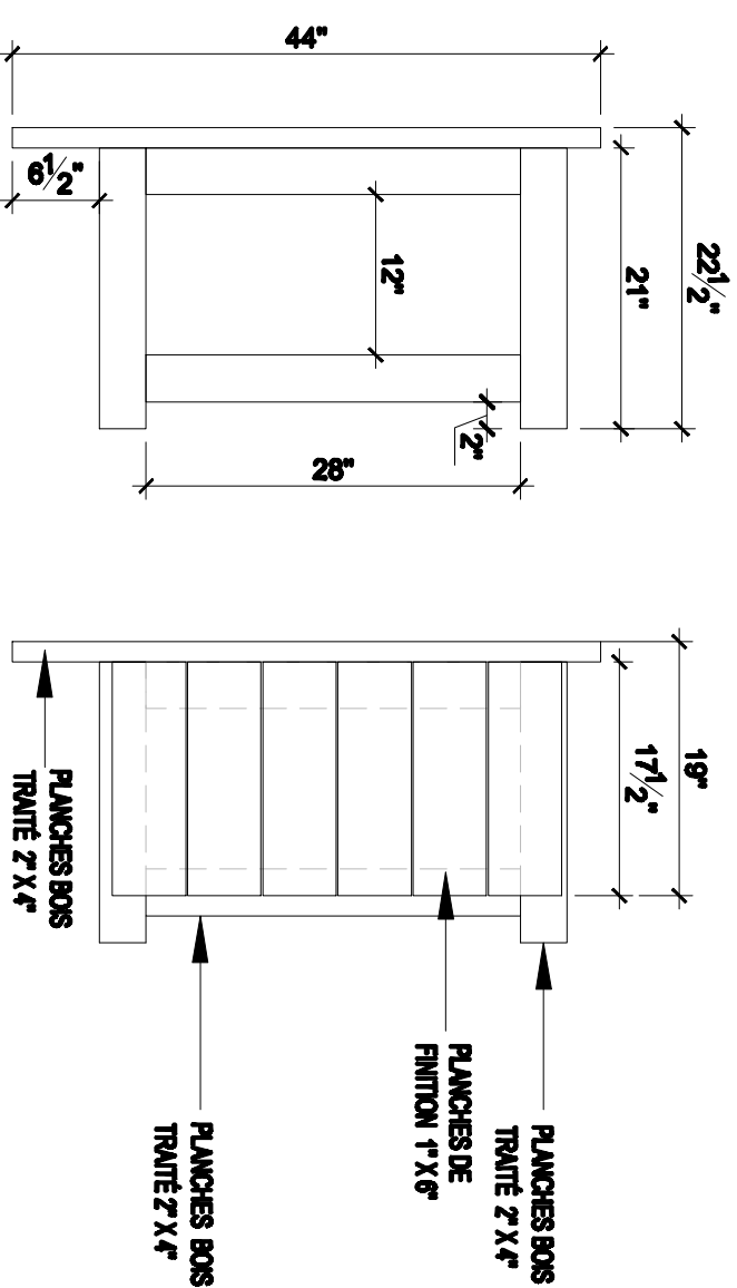
ÉLEVATION C CÔTÉ
